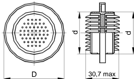
Эскиз – ПМ1
