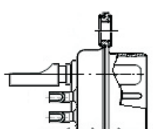
Вилка РП15 объемного монтажа с силовыми Вставками Стр. 14
