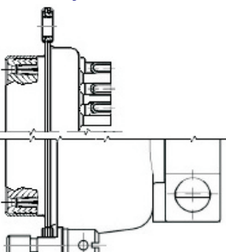
Розетка РП15 объемного монтажа без кожухом
