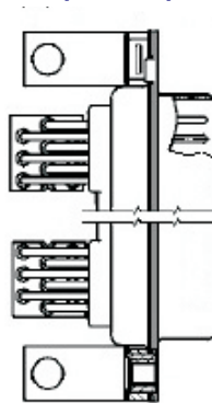
Вилка РП15 углового печатного монтажа без фиксатора
