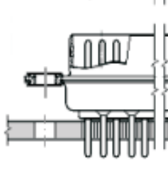
Вилка РП15 печатного монтажа без фиксатора
