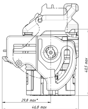
СНК-1-32РОЗ-0602
