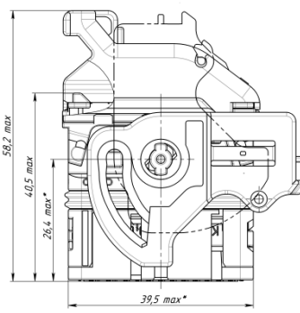
СНК-2-48РОЗ-0201
