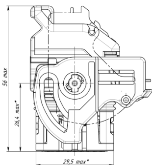
СНК-1-32РОЗ-0601
