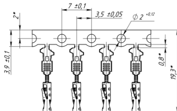
СНК-1-32РОЗ-0602
