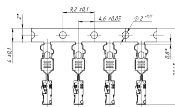
СНК-2-48РОЗ-0202
