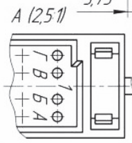
Розетки ГСНП58А-72РП21, ГСНП58А-72РП22
