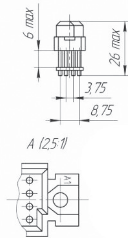
Розетки ГСНП58А-72РП21, ГСНП58А-72РП22
